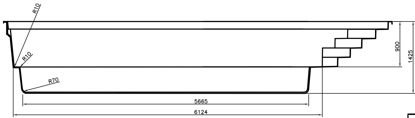
Doorsnede A-A
